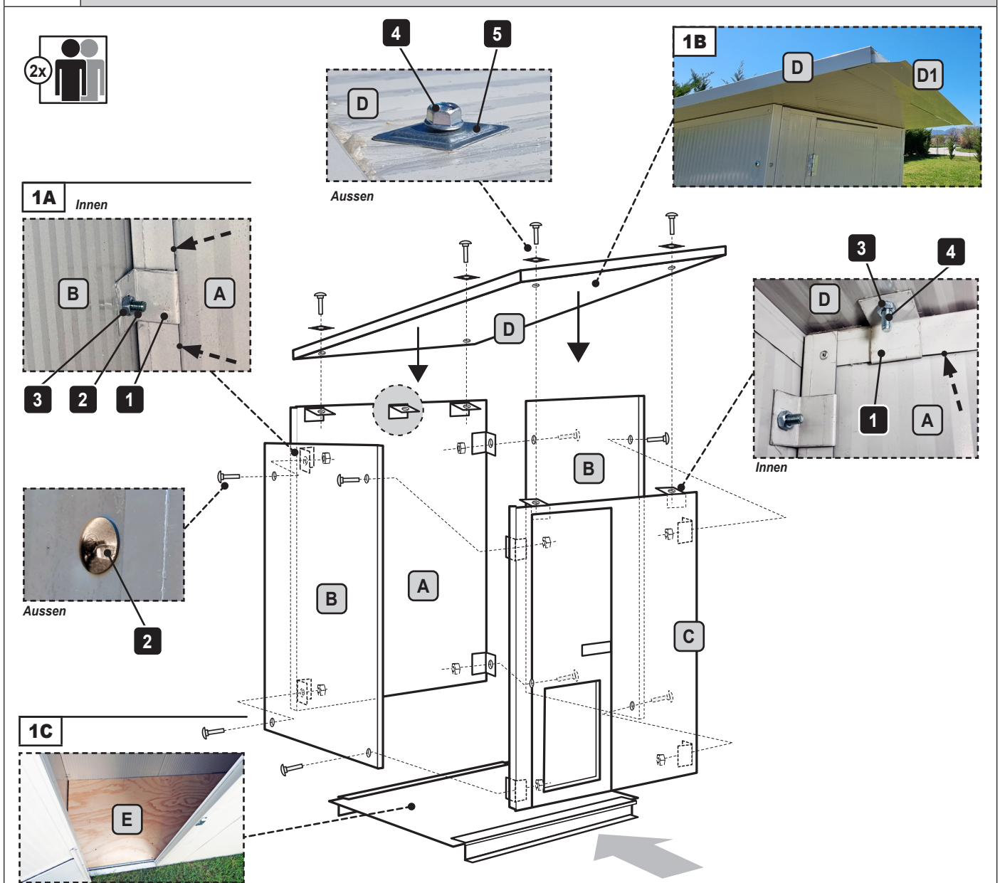
Abb. 1 MONTAGEPLAN DER HUNDEHÜTTE
